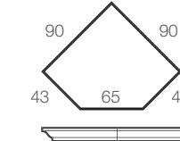
667/T Cappello / Frame H. 7
