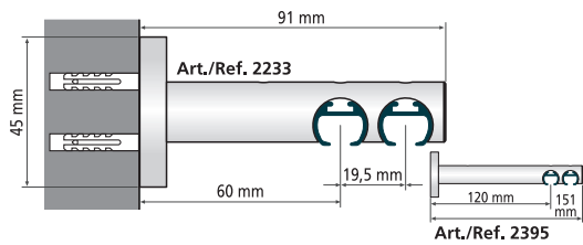
SUPPORTO 2 CANALI / 2 WAYS SUPPORT
